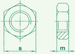
DIN 934
