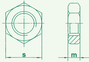
DIN 439
